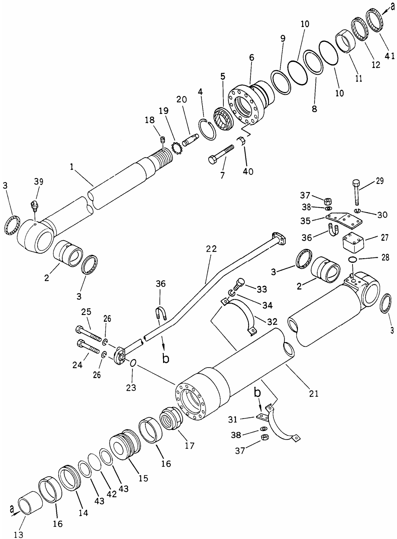
FIG: 6140 ARM CYLINDER
