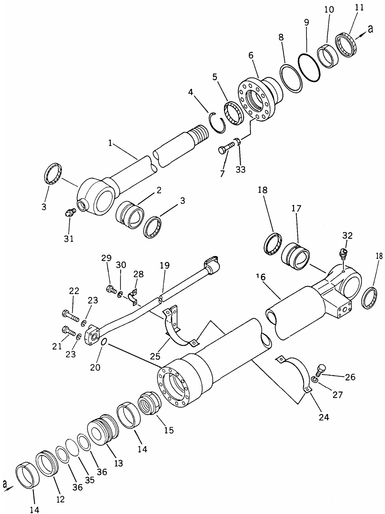
FIG: 6150 BUCKET CYLINDER
