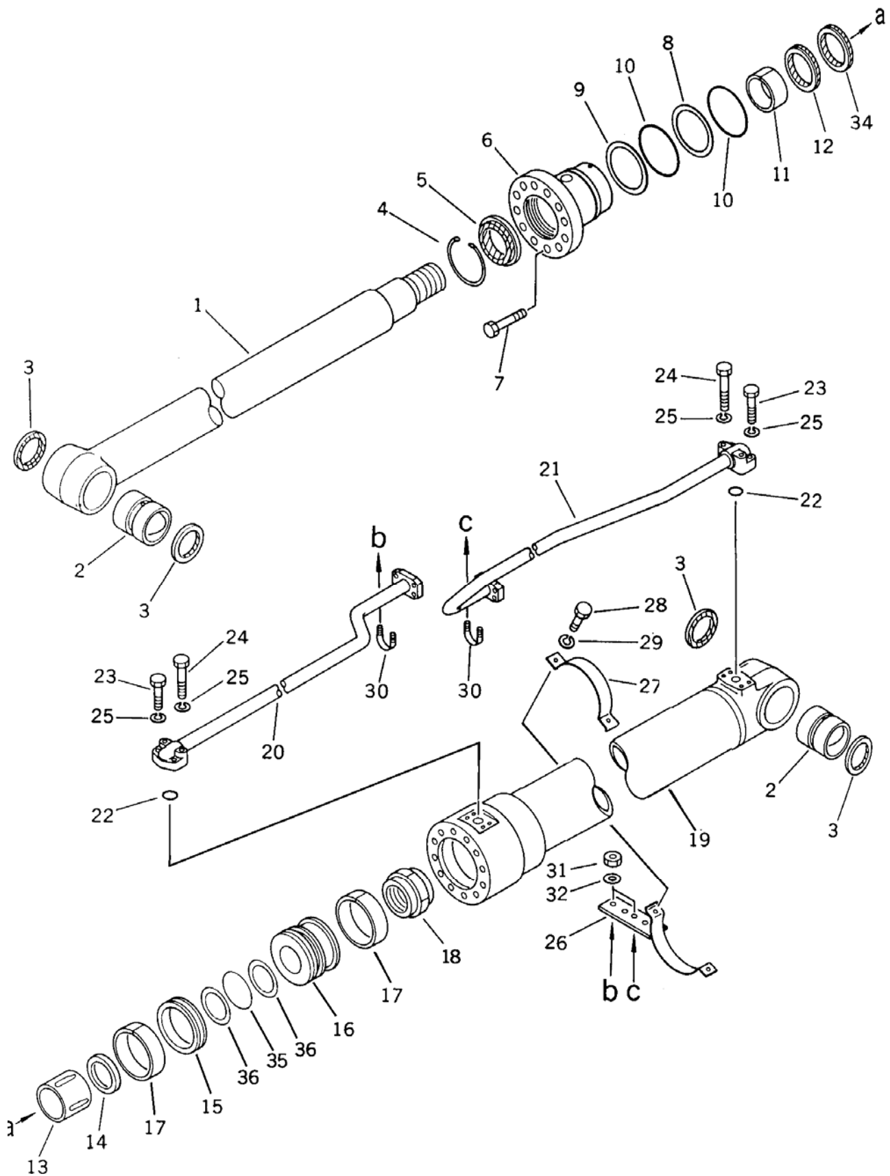
FIG: 6130 BOOM CYLINDER
